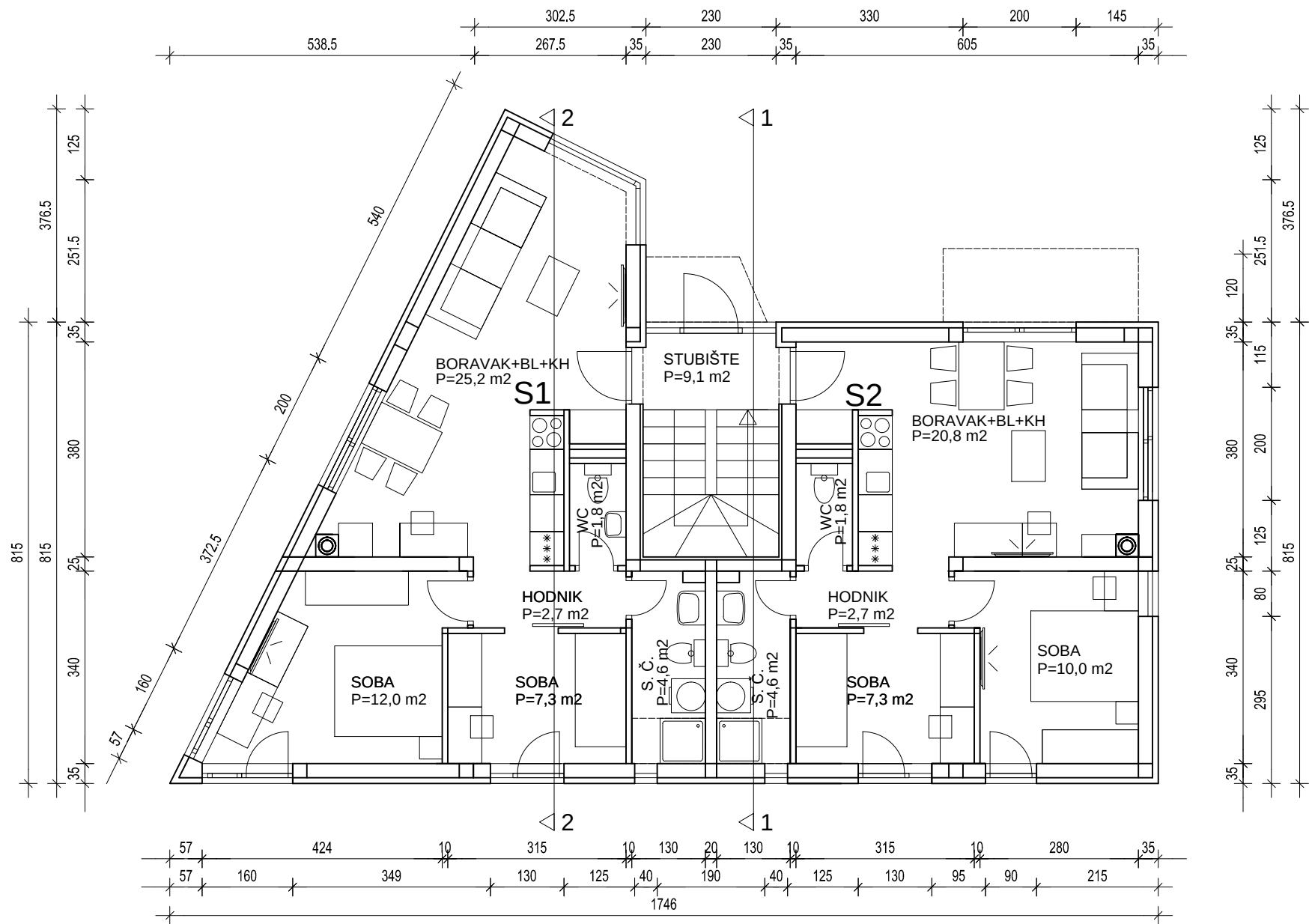
TLOCRT PRIZEMPLJA 1:100
