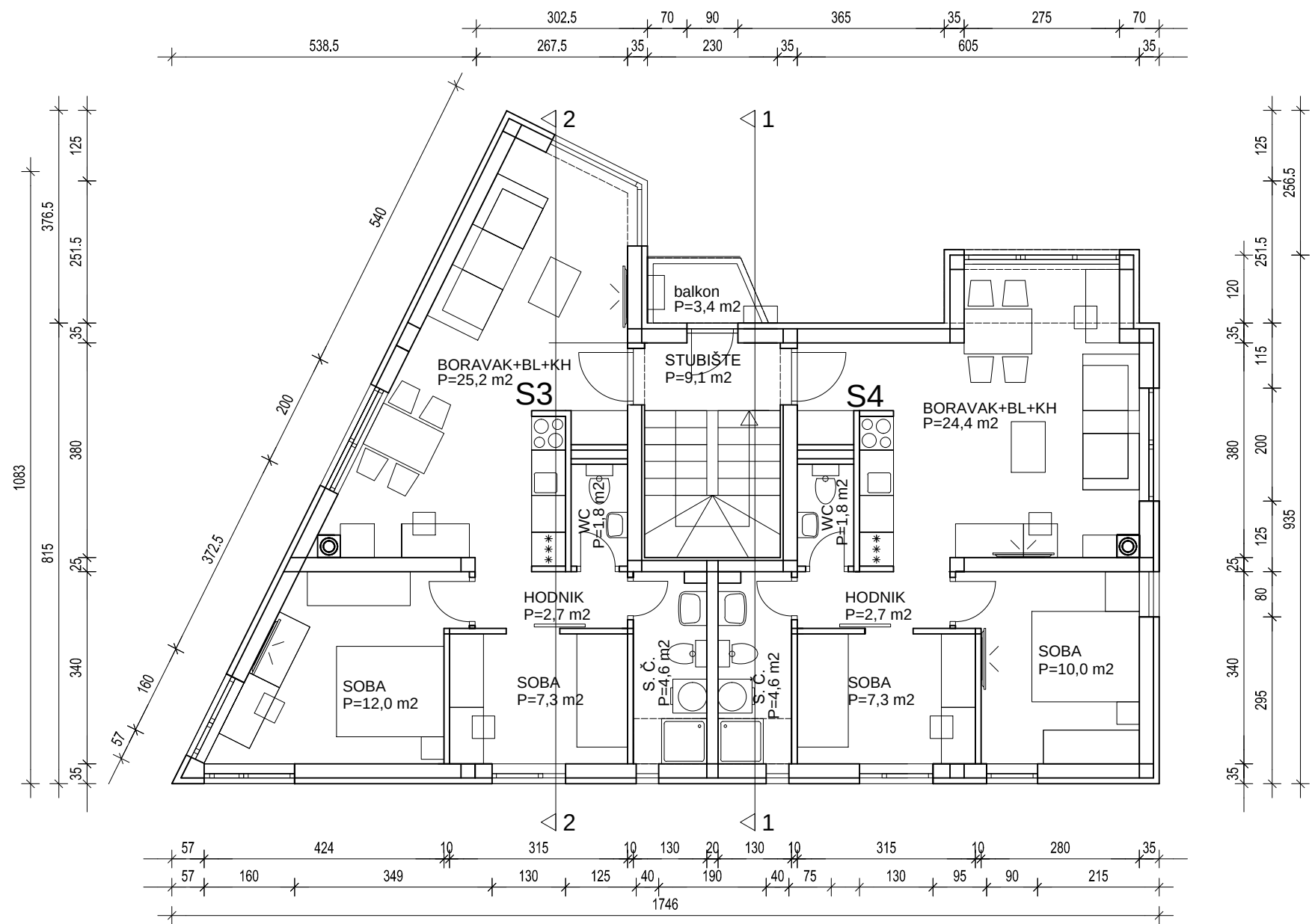
TLOCRT I KATA 1:100
