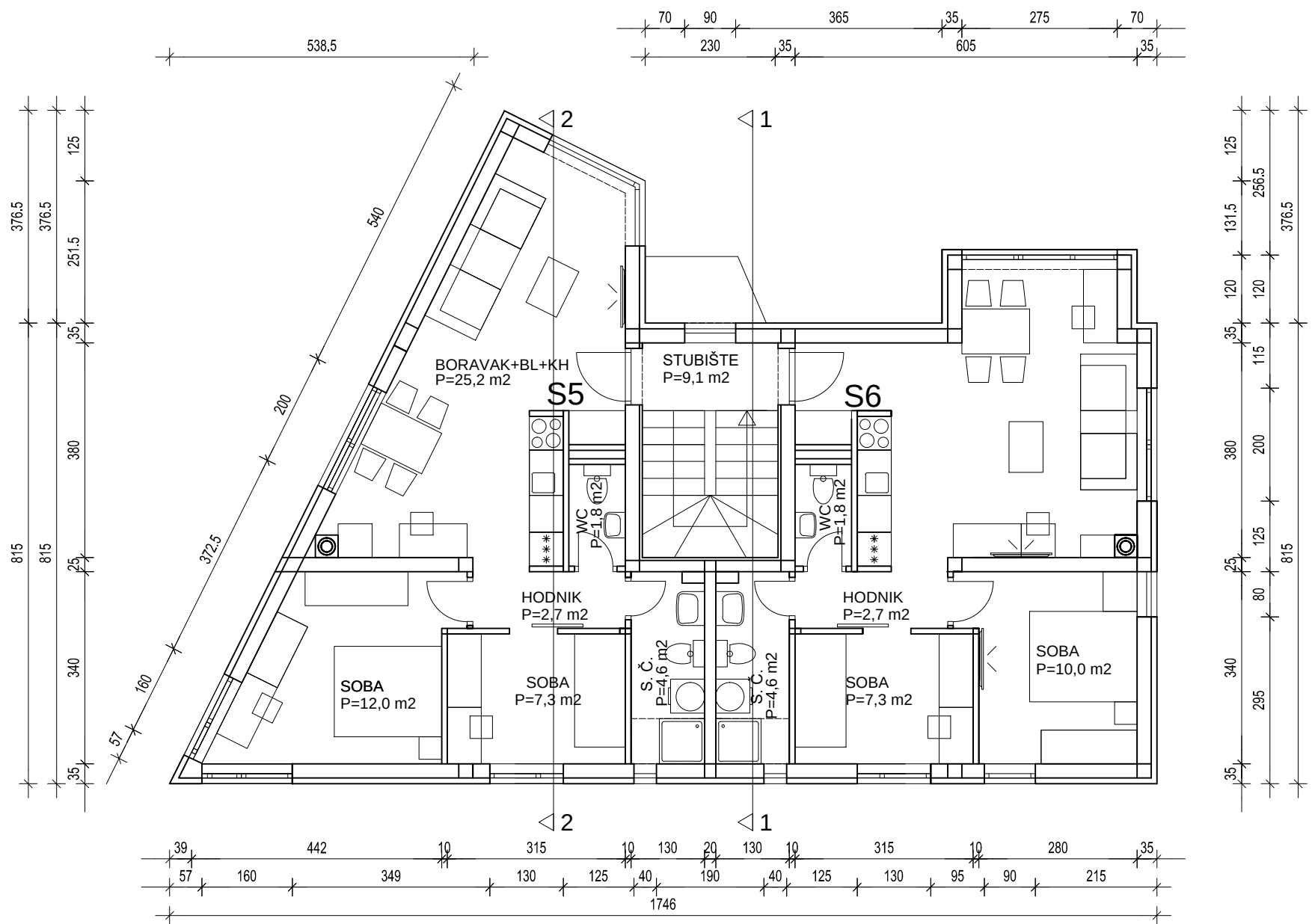
TLOCRT II KATA 1:100
