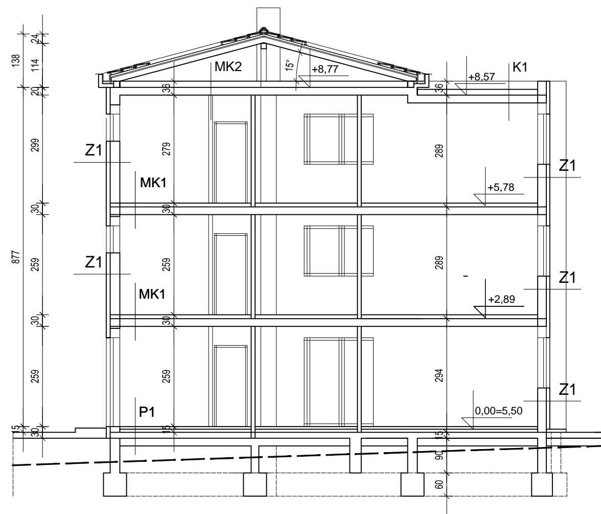
PRESJEK 2-2 1:100
