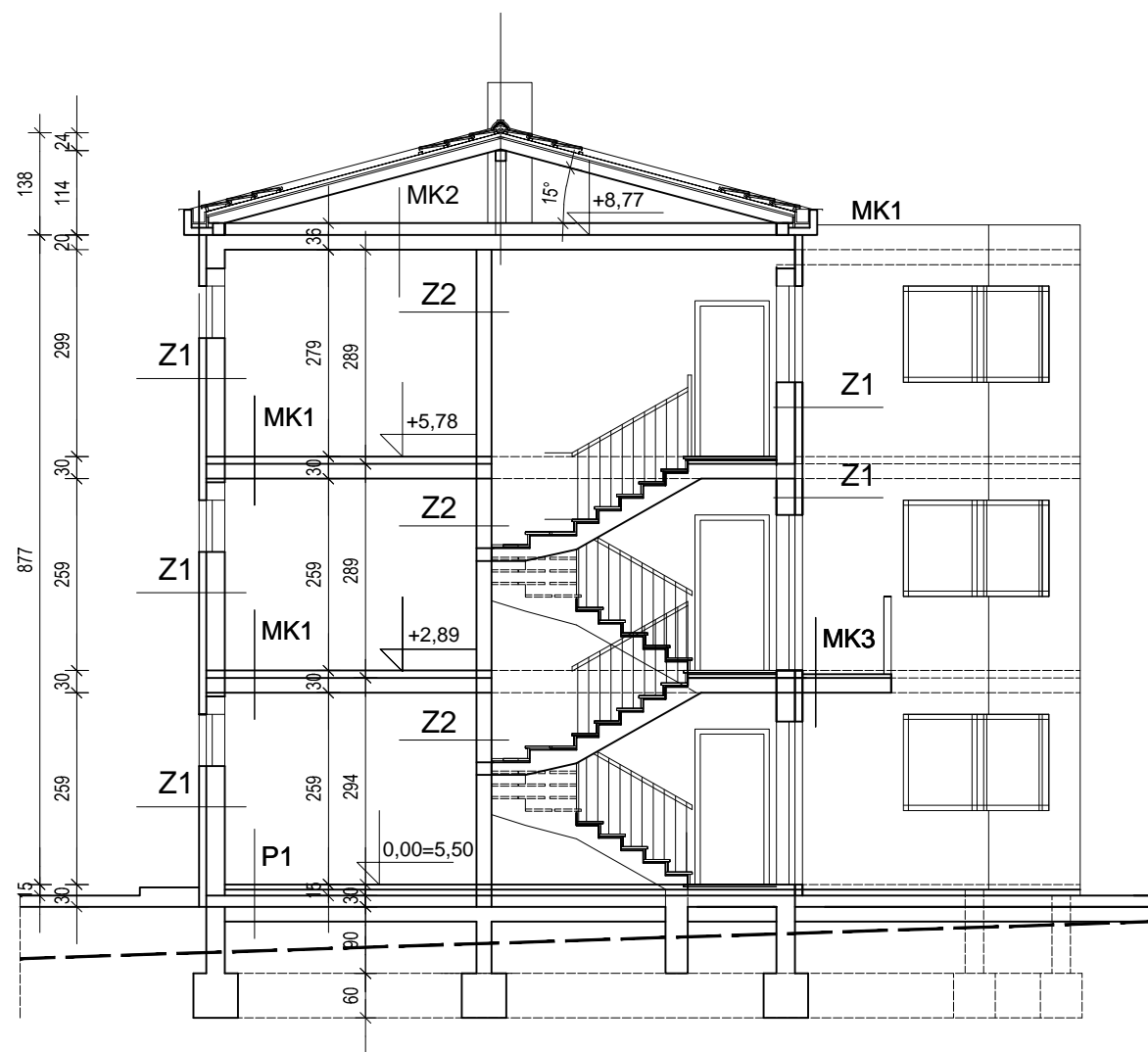
PRESJEK 1-1 1:100
