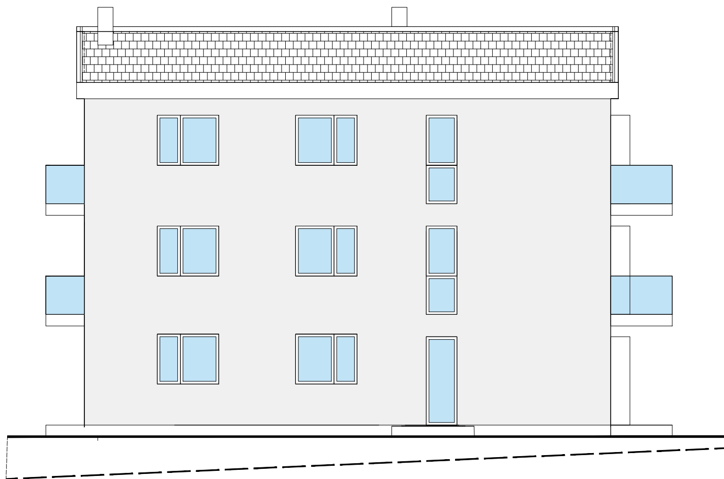
JUGOISTOČNO PROČELJE 1:100
