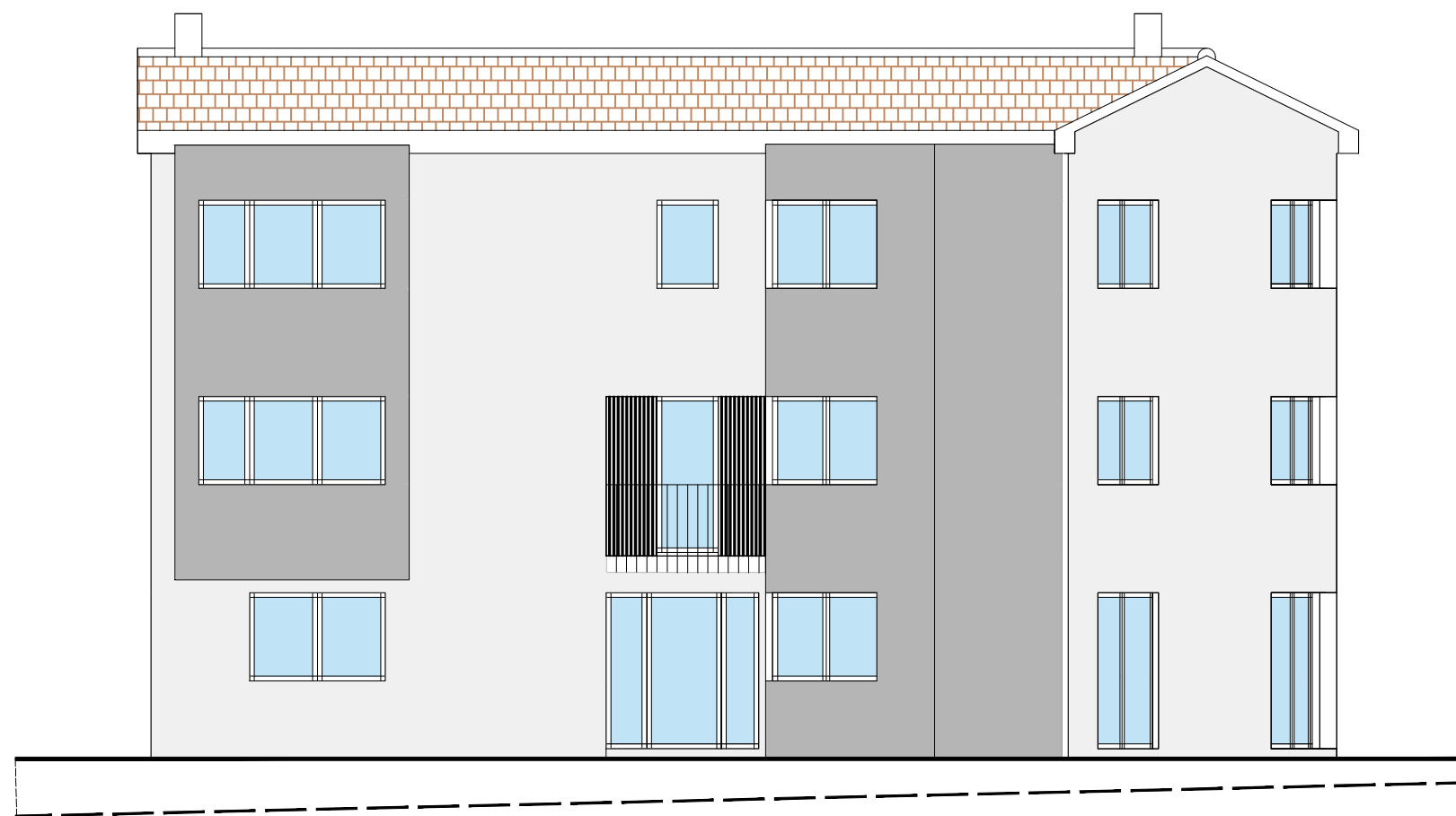
SJEVEROISTOČNO PROČELJE 1:100
