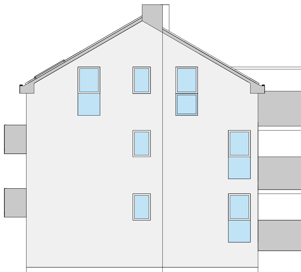
SJEVEROZAPADNO PROČELJE 1:100
