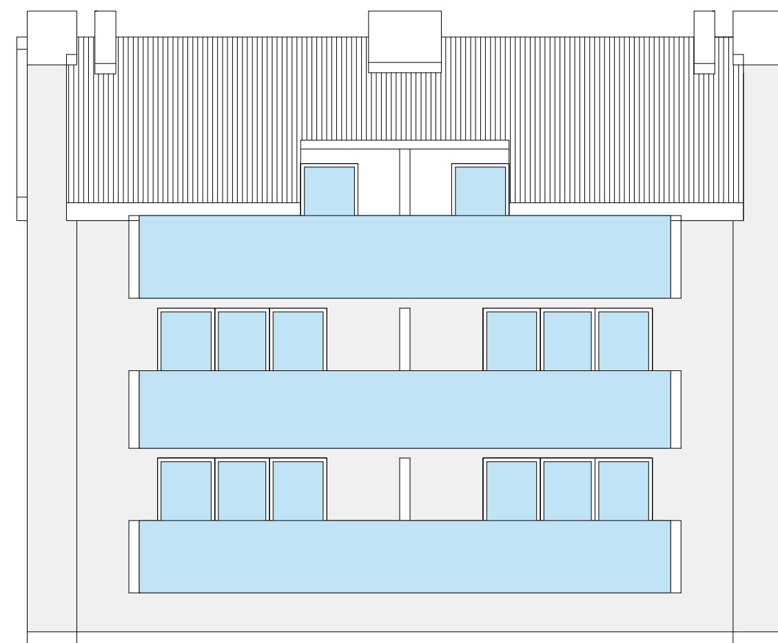
JUGOZAPADNO PROČELJE 1:100
